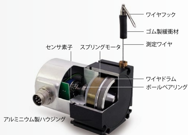
WDS-P60を例にしたセンサ構造
