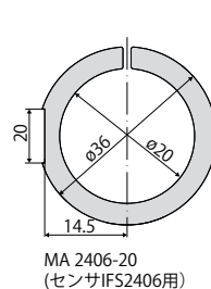
取付リング
