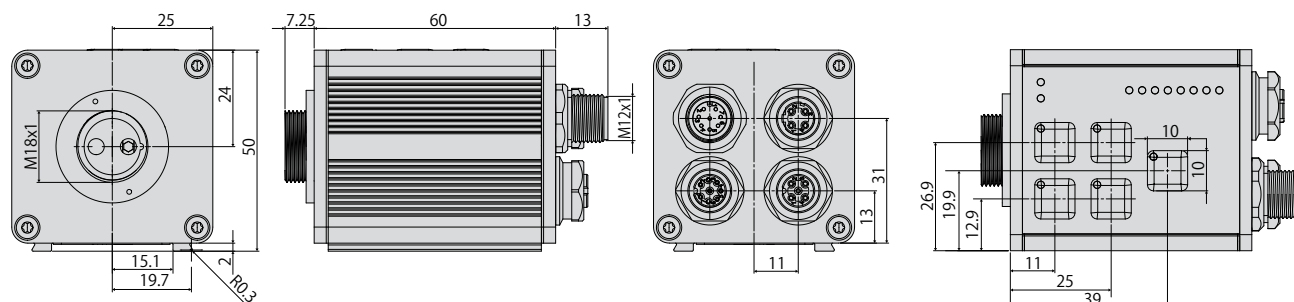
外径寸法: 単位はmm、図は縮尺通りではない
