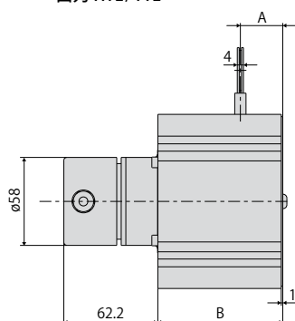
出力 HTL/TTL
