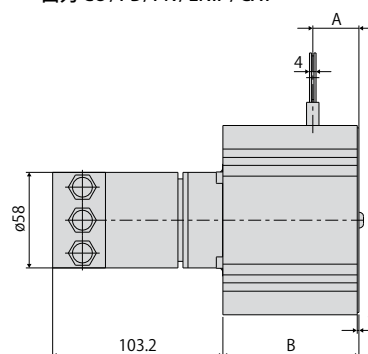
出力 CO/PB/PN/ENIP/CAT
