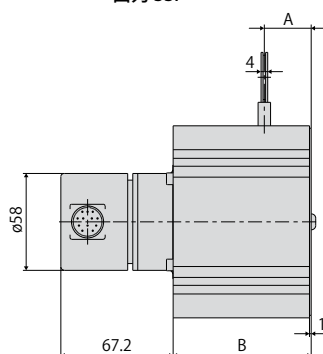
出力 SSI
