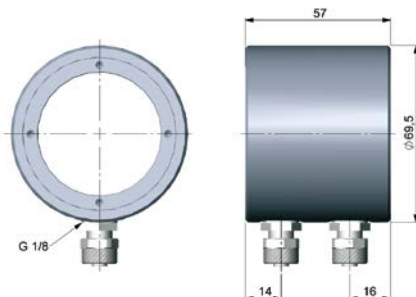
TM-W-CTL Wasserkühlgehäuse
