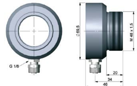
TM-AP-CTL Freiblasvorsatz
