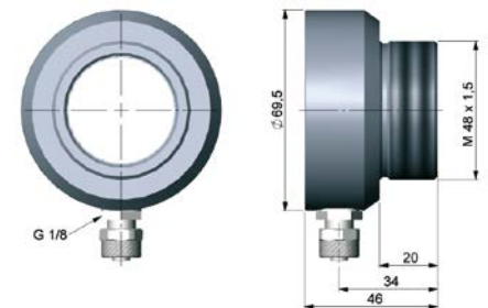
TM-AP-CTL Dispositif de soufflage
