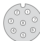
8ピンのハウジングコネクタ M12x1 ピン側から見た図
