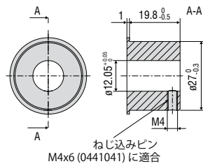
センサホルダ JMA-12用
