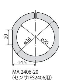
取付リング
