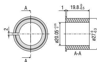
センサホルダ JMA-20用
