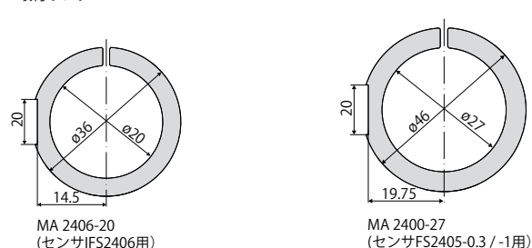
取付リング
