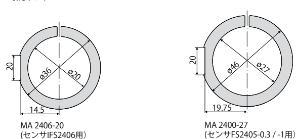
取付リング
